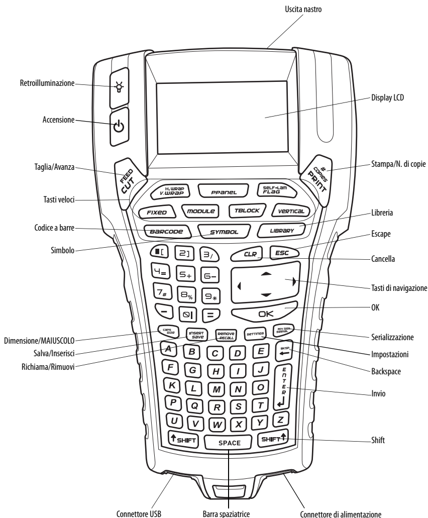
Figura 1 Stampante RHINO 6000
