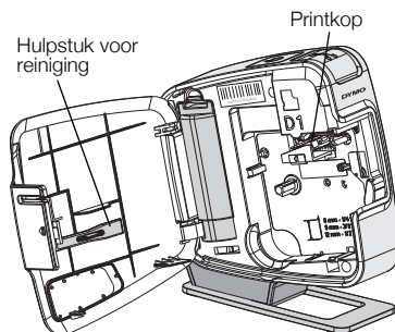
Afbeelding 7
